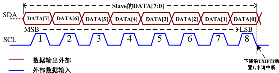
SLAVE的8+0发送模式: SIMODE[2:0]=111
