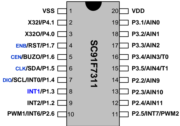
SC91F7311管脚配置图
