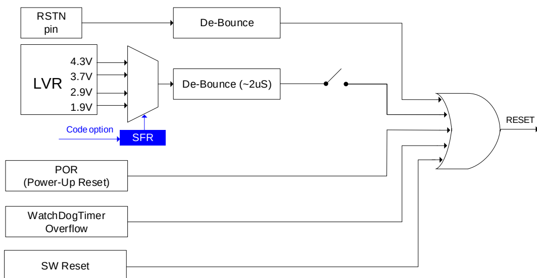
SC95FWXX 复位电路图
