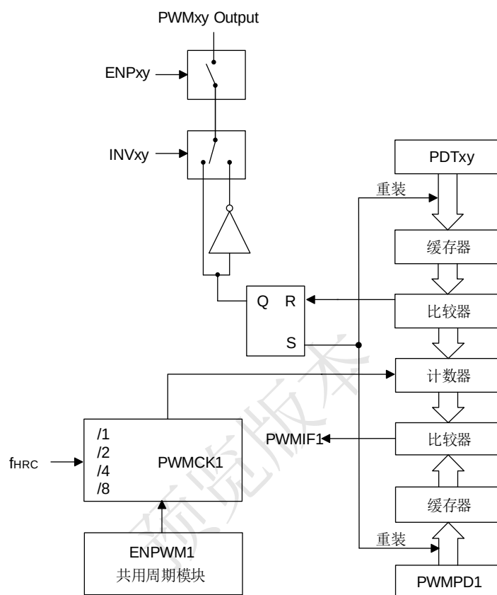
SC95FWXX PWM1 独立模式框图
