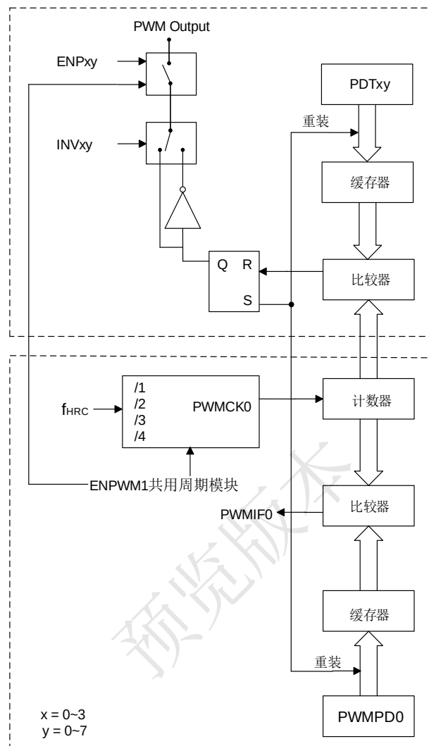
SC95FWXX PWM0 结构框图
