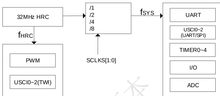
SC95FWXX 内部时钟关系
