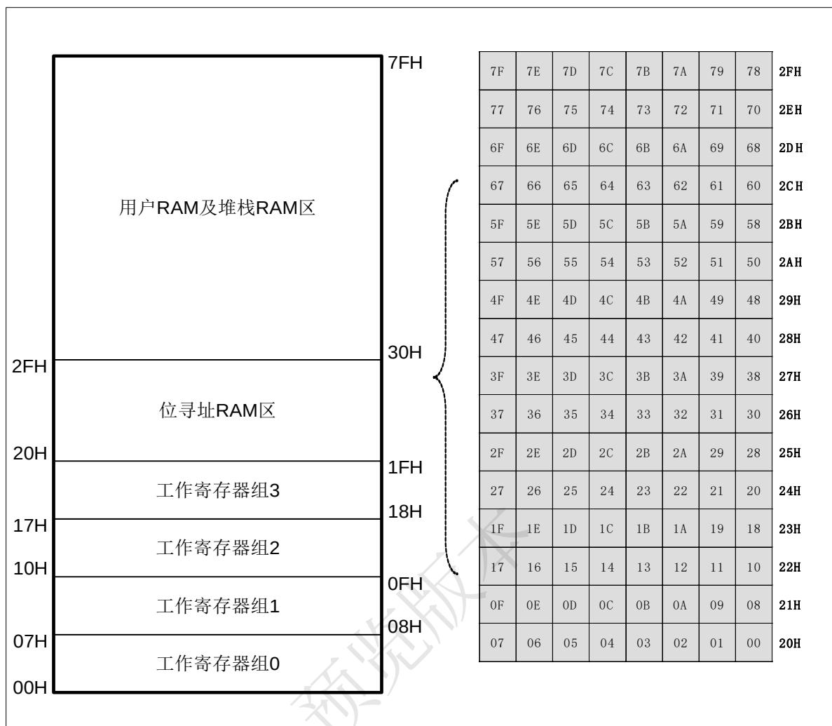
SRAM 结构图
