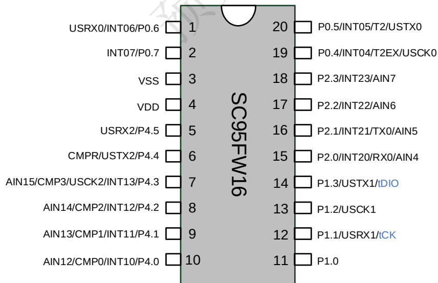
SC95FW16 管脚配置图
