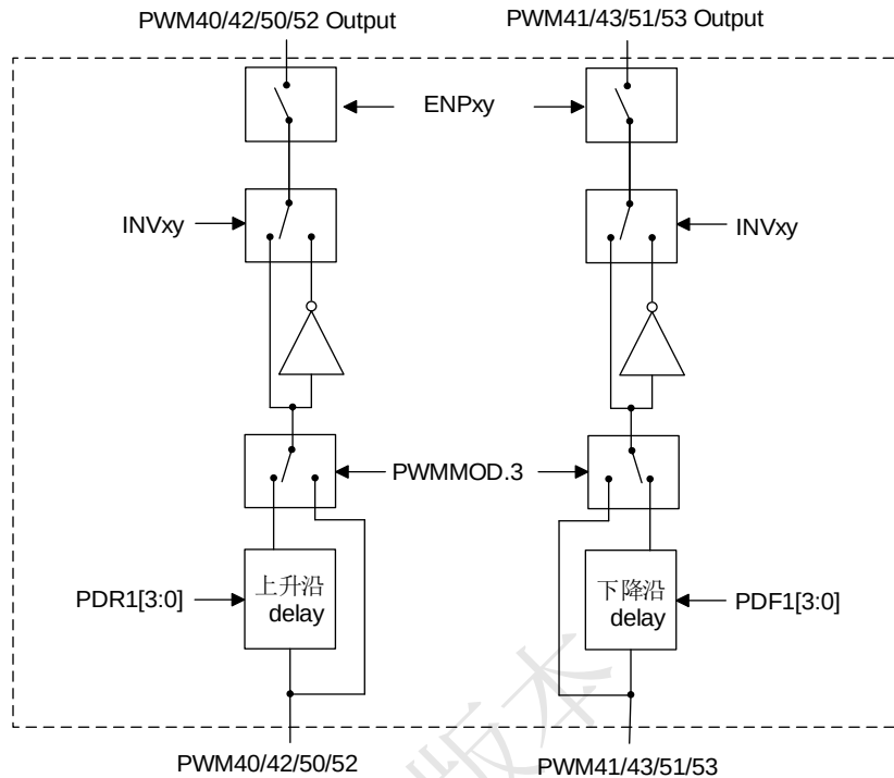
SC95FWXX PWM 互补模式框图
