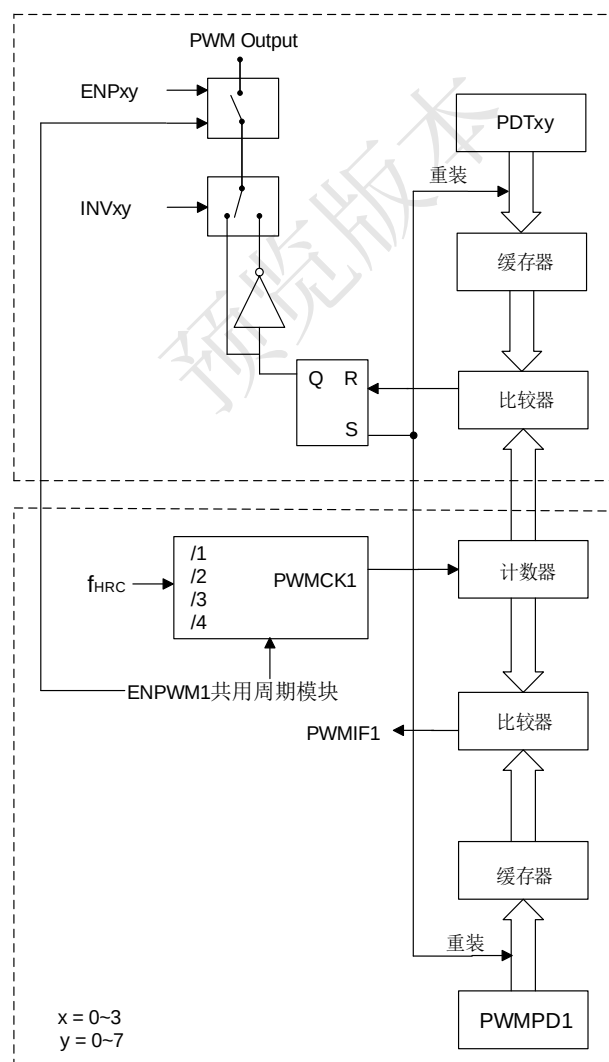
SC95FWXX PWM1 结构框图
