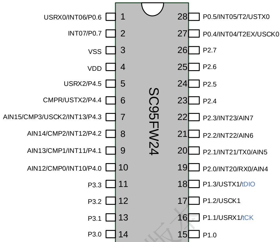
SC95FW24 管脚配置图
