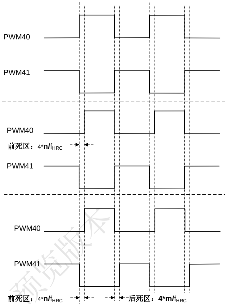
PWM1 死区输出波形
