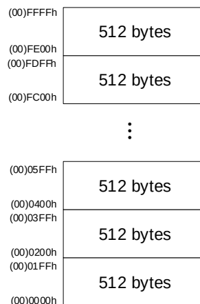
SC95FWXX 64 Kbytes Flash ROM Sector 分区示意
