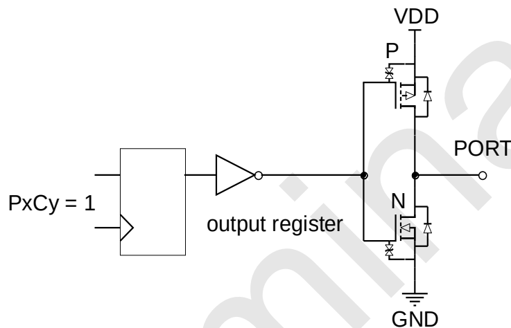
强推挽输出模式
