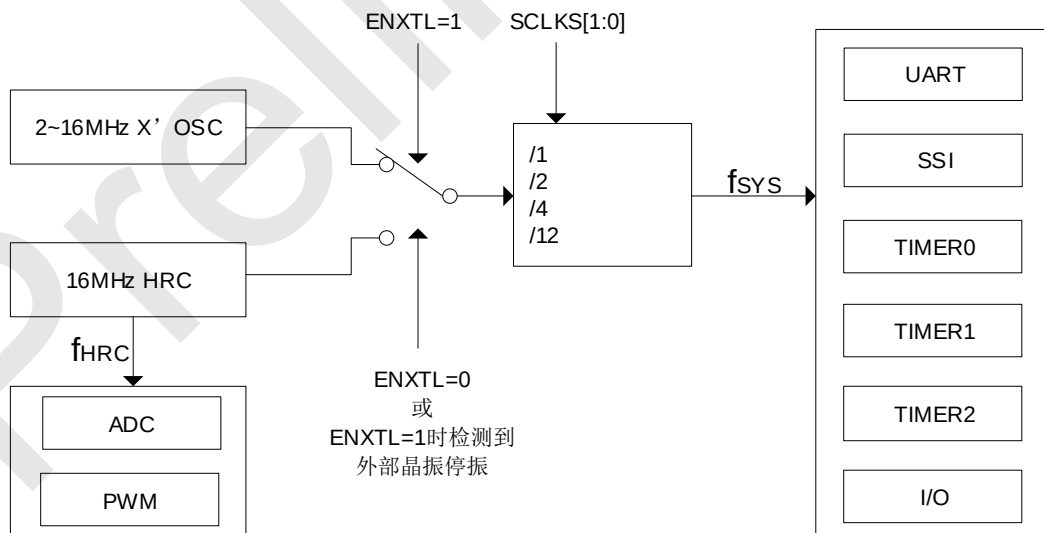
SC92F8003B 内部时钟关系
