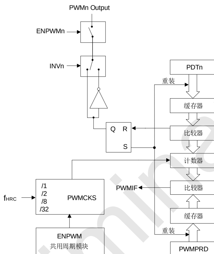
SC92F8003B PWM 独立模式框图
