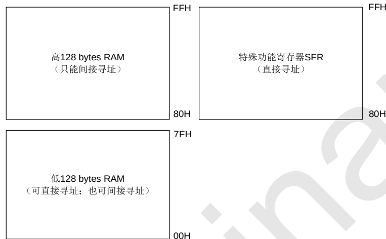
内部 256 bytes RAM 结构图
