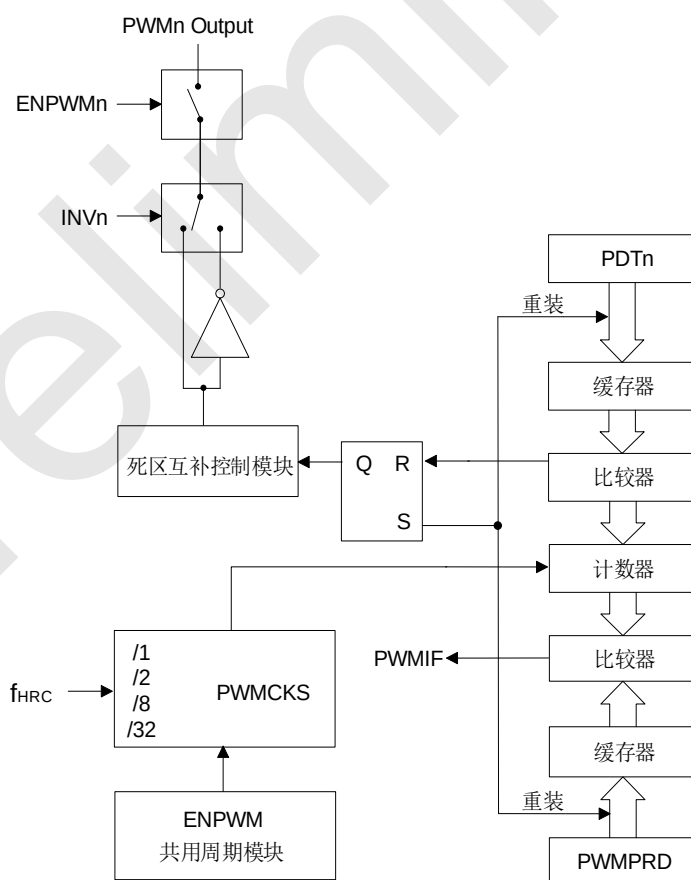
SC92F8003B PWM 结构框图
