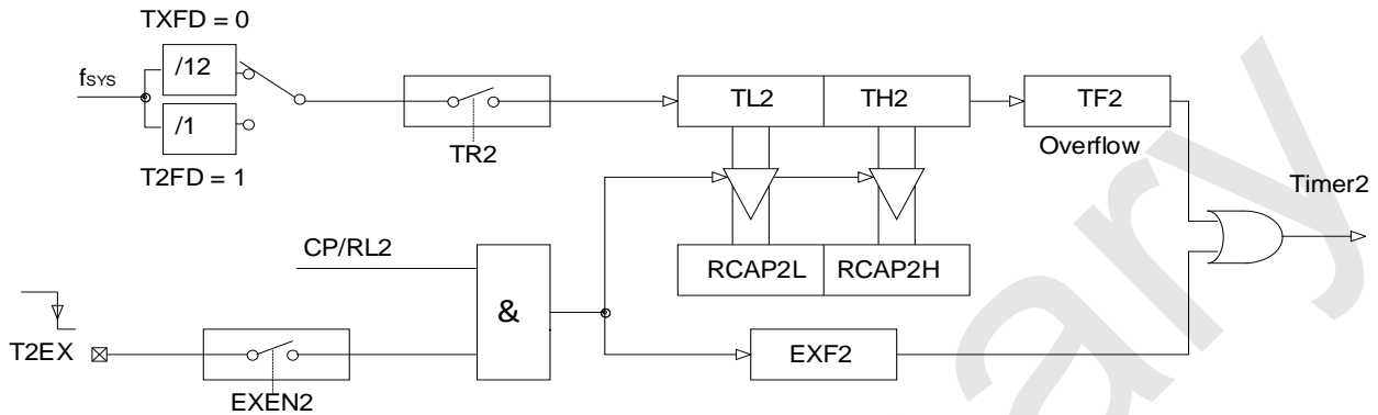
模式 0：16 位捕获
