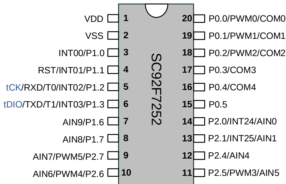
SC92F7252 管脚配置图 (TSSOP20、SOP20)
