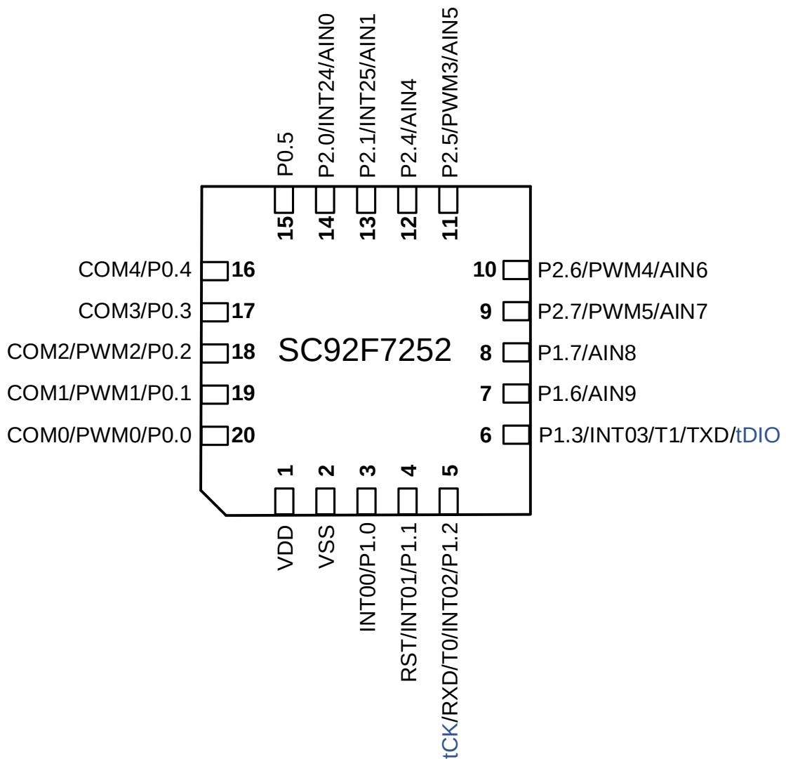
SC92F7252 管脚配置图 (QFN20)
