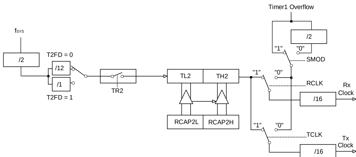
模式 2：波特率发生器
