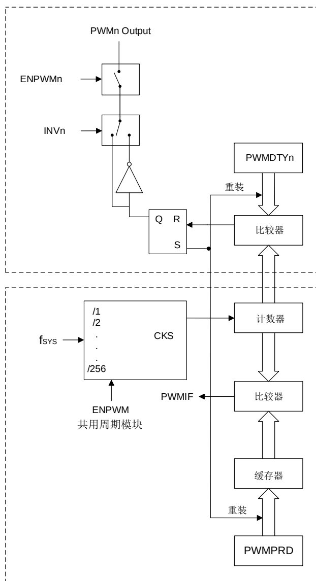
SC92F725X PWM 结构框图
