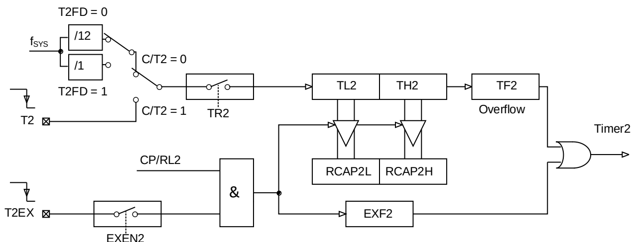
模式 0：16 位捕获
