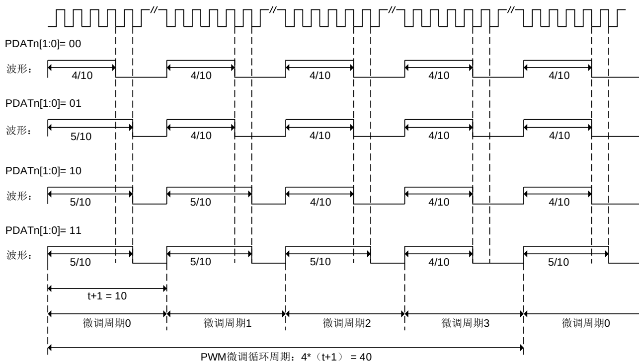
8+2 位 PWM 微调控制示意图
