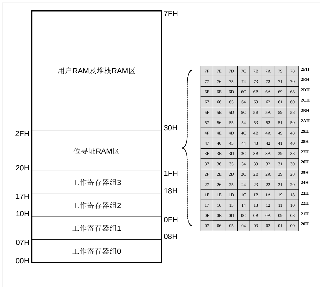
SRAM 结构图
