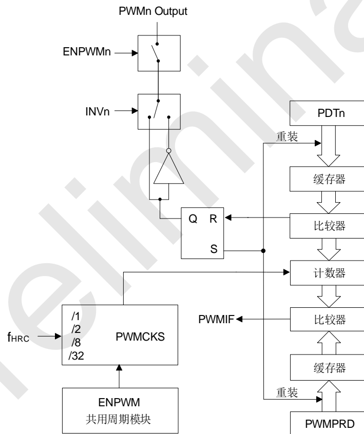
SC92F740X PWM 独立模式框图
