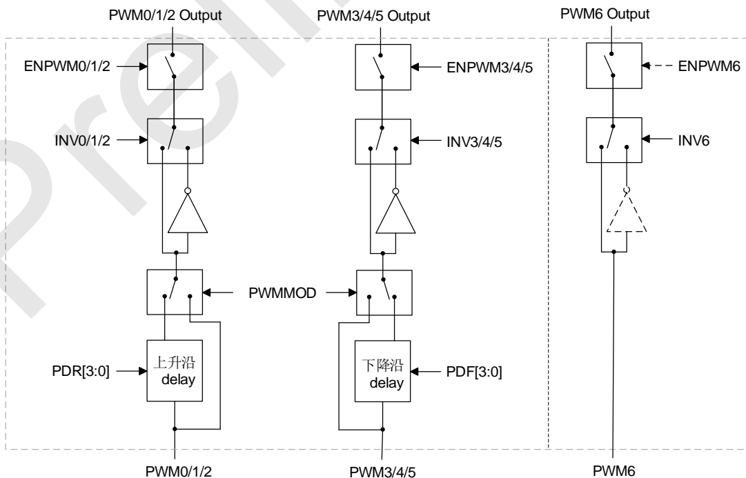
SC92F740X PWM 互补模式框图
