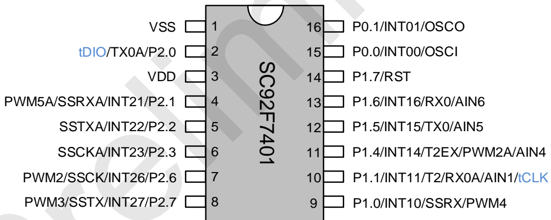
SC92F7401 管脚配置图
