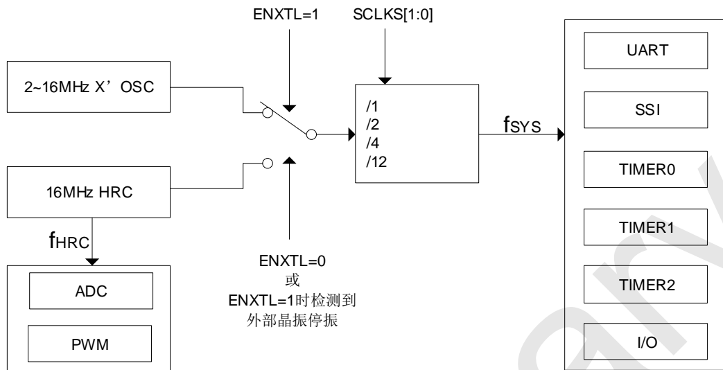
SC92F740X 内部时钟关系
