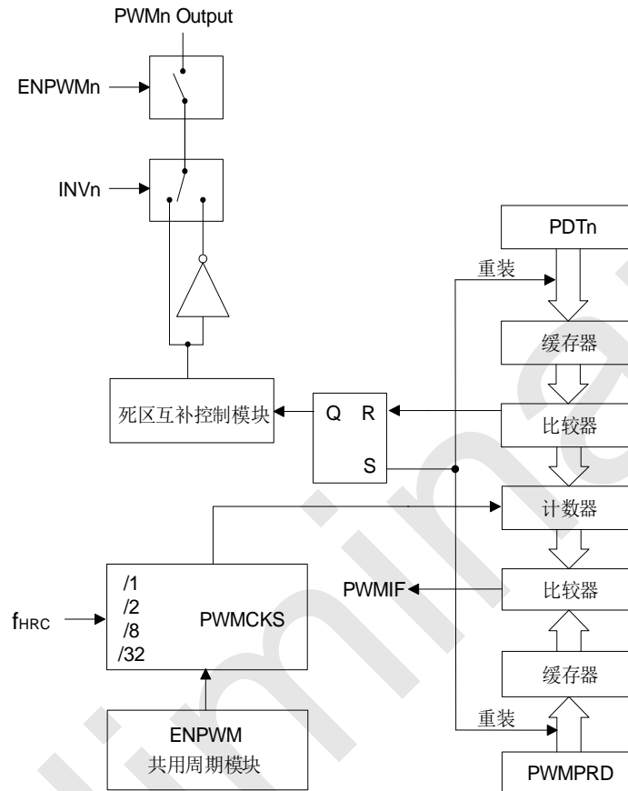
SC92F740X PWM 结构框图
