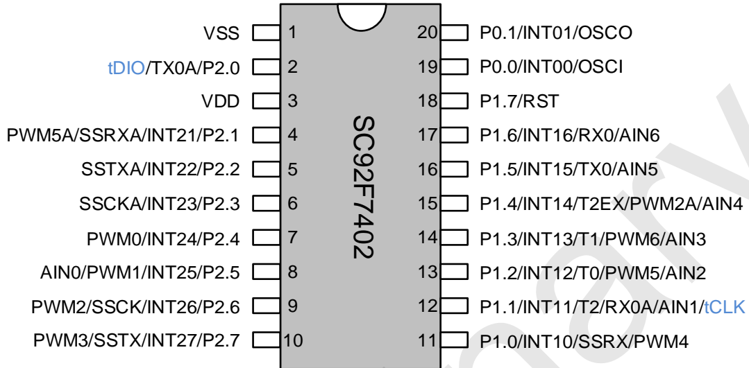
SC92F7402 管脚配置图
