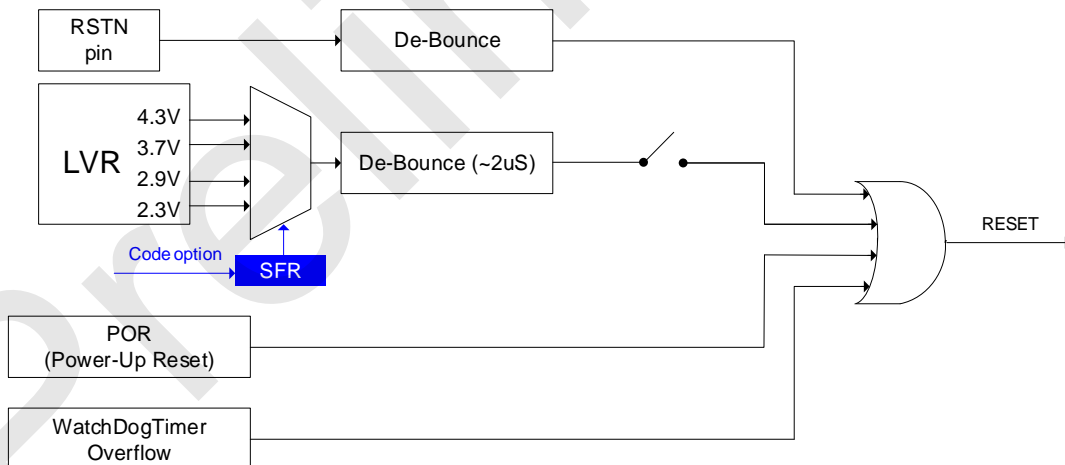
SC92F740X 复位电路图
