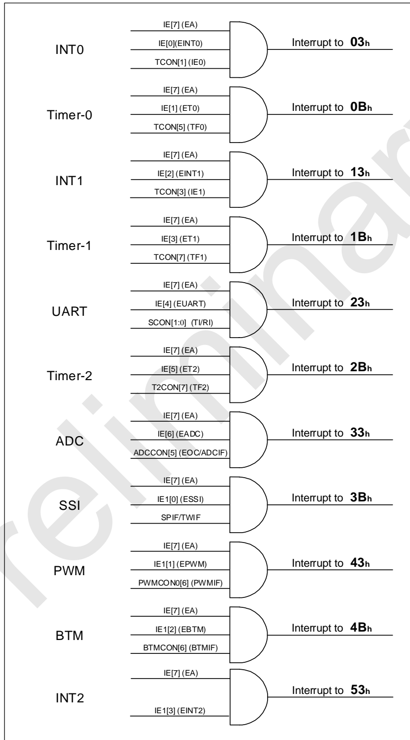
SC92F740X 中断结构和向量
