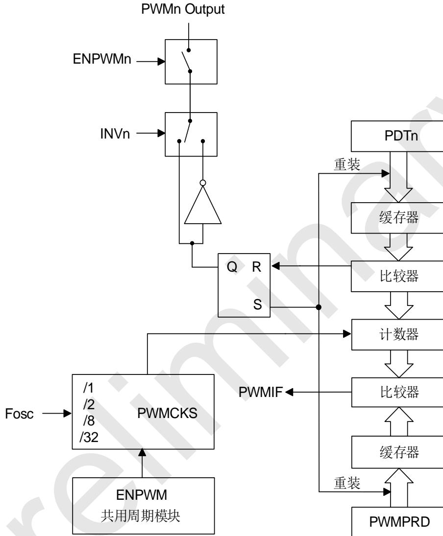
SC92F84AX PWM 独立模式框图
