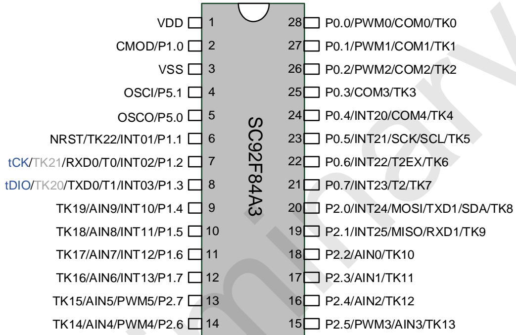
SC92F84A3 管脚配置图
