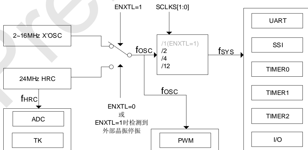
SC92F84AX 内部时钟关系
