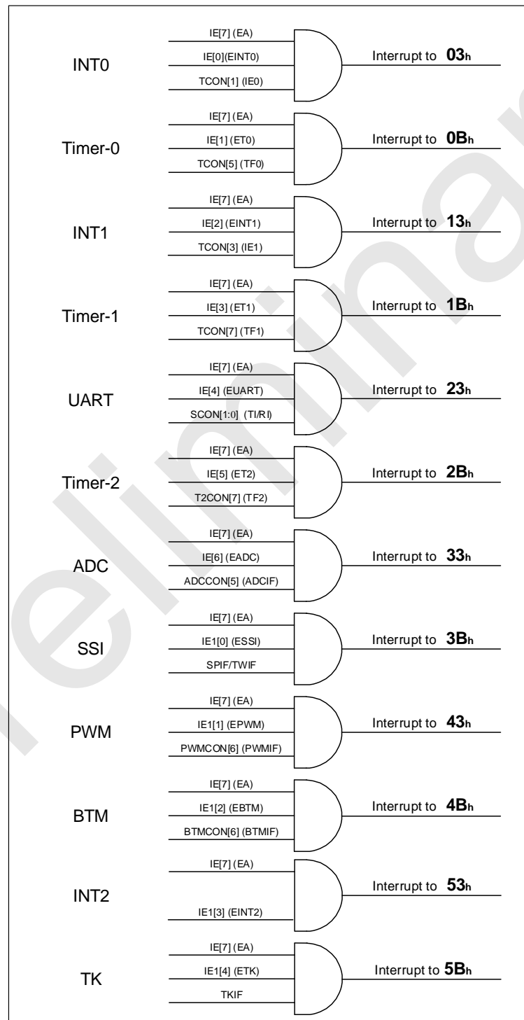
SC92F84AX 中断结构和向量
