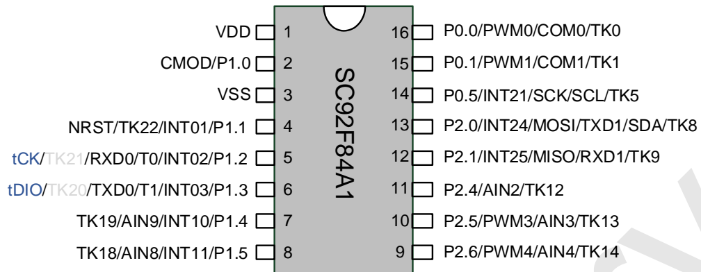
SC92F84A1 管脚配置图
