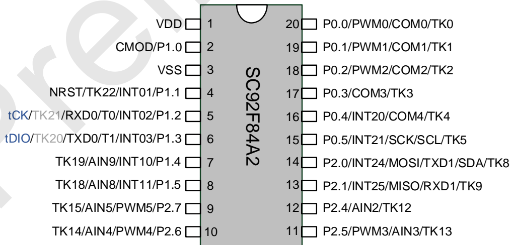
SC92F84A2 管脚配置图
