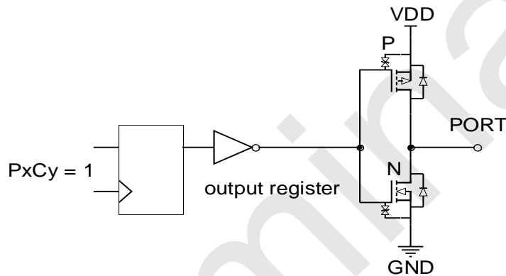
强推挽输出模式
