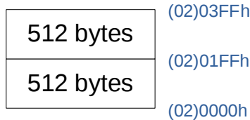
SC92L753X EEPROM Sector 分区示意
