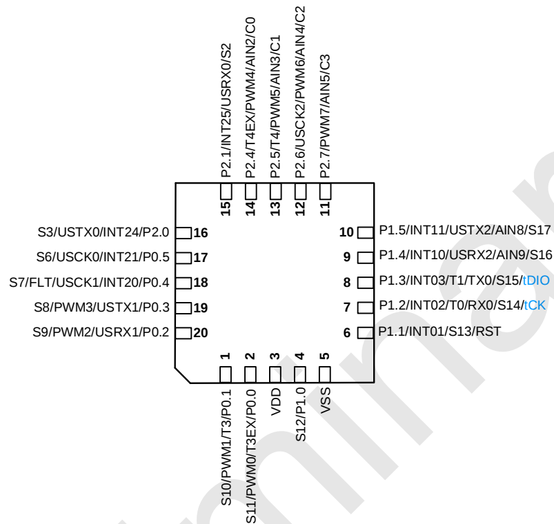
SC92L7532 管脚配置图 (QFN20 3*3)
