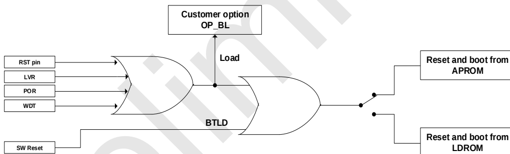
SC92L753X 复位后启动区域切换示意图
