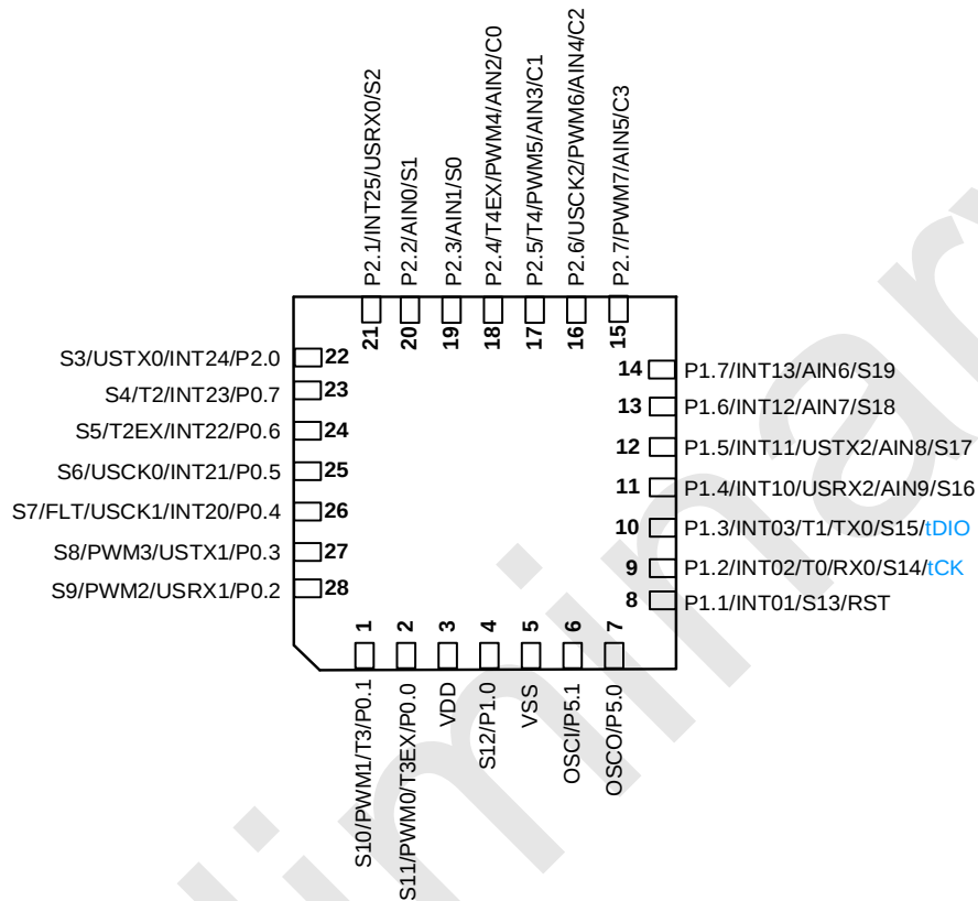
SC92L7533 管脚配置图 (QFN28 4*4)
