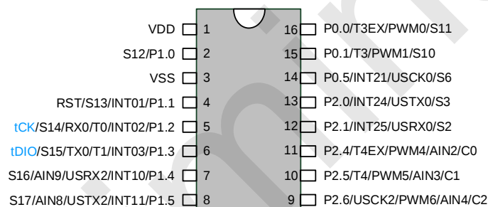
SC92L7531 管脚配置图 (SOP16)
