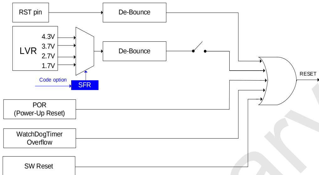
SC92L753X 复位电路图
