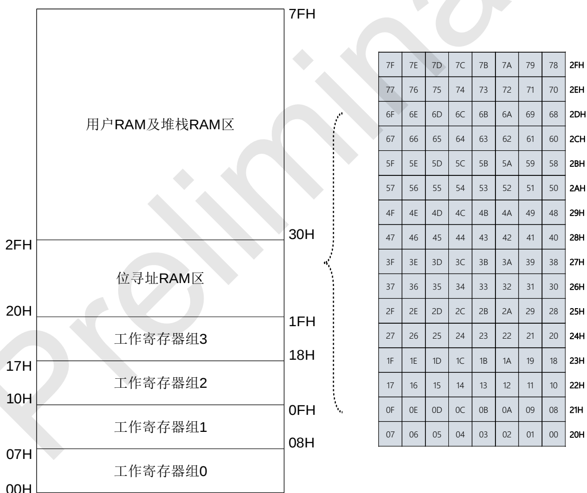
SRAM 结构图
