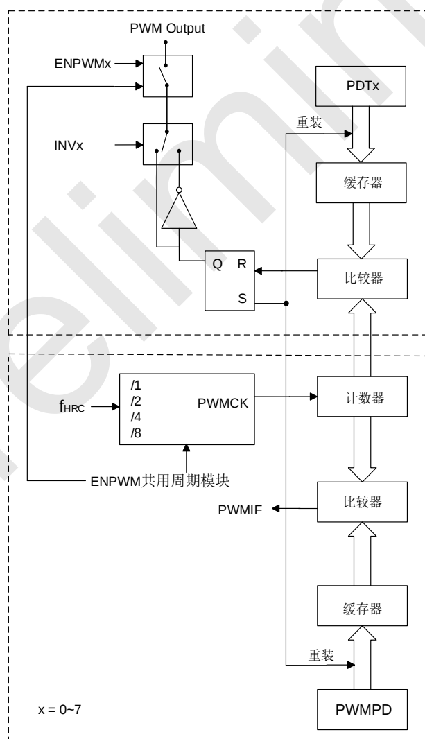
SC92L753X PWM 结构框图
