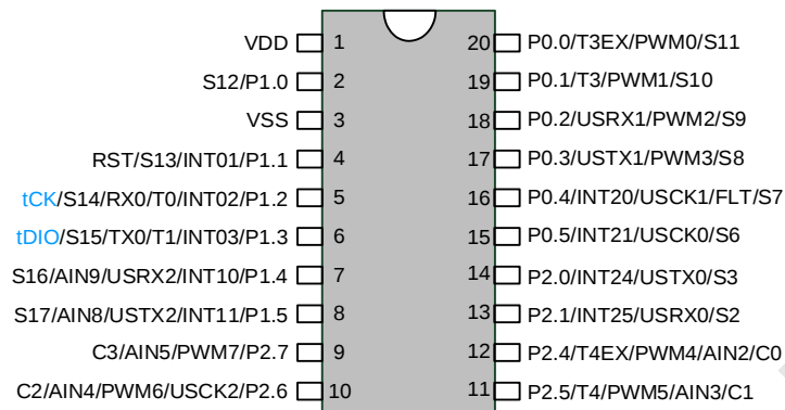
SC92L7532 管脚配置图 (SOP20/TSSOP20)
