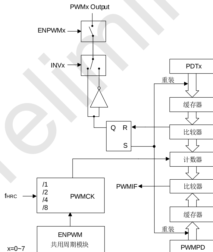
SC92L753X PWM 独立模式框图
