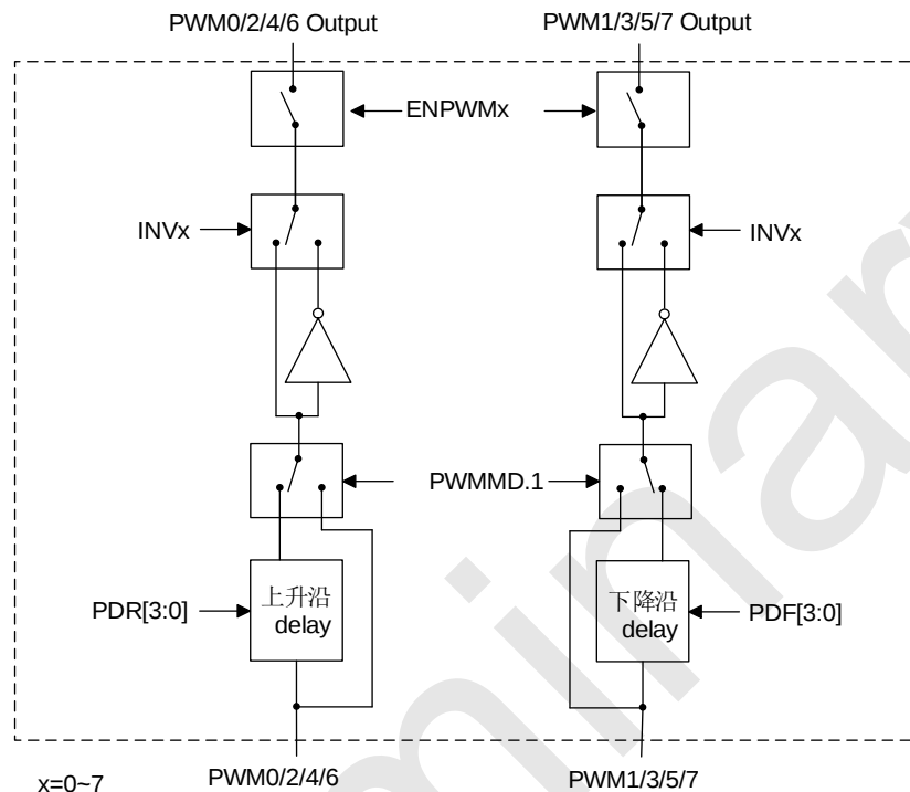
SC92L753X PWM 互补模式框图
