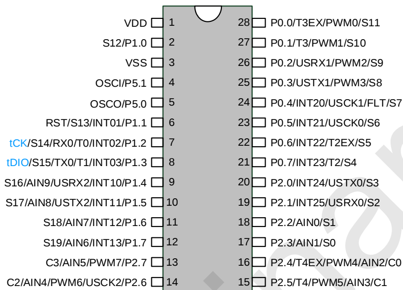
SC92L7533 管脚配置图 (SOP28/TSSOP28)
