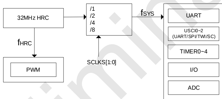
SC92L753X 内部时钟关系
