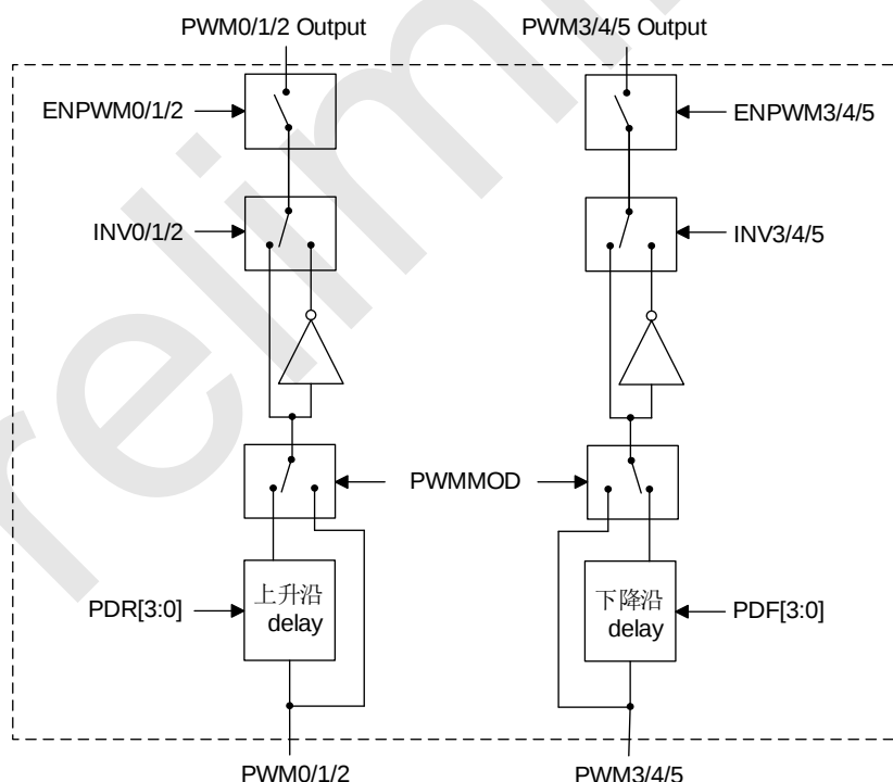
SC92R425 PWM 互补模式框图
