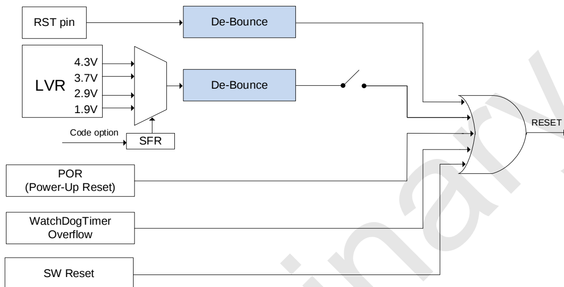
SC92R425 复位电路图
