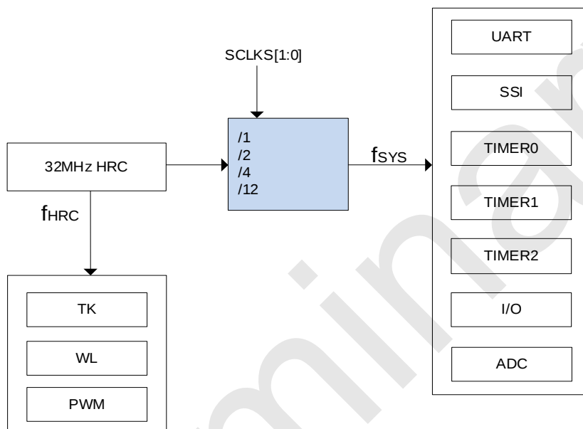
SC92R425 内部时钟关系
