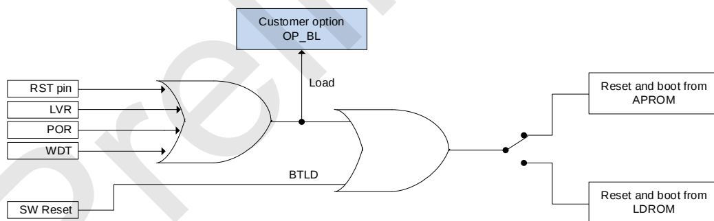
SC92R425 复位后启动区域切换示意图
