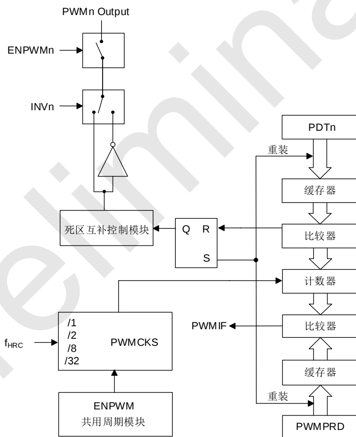
SC92R425 PWM 结构框图
