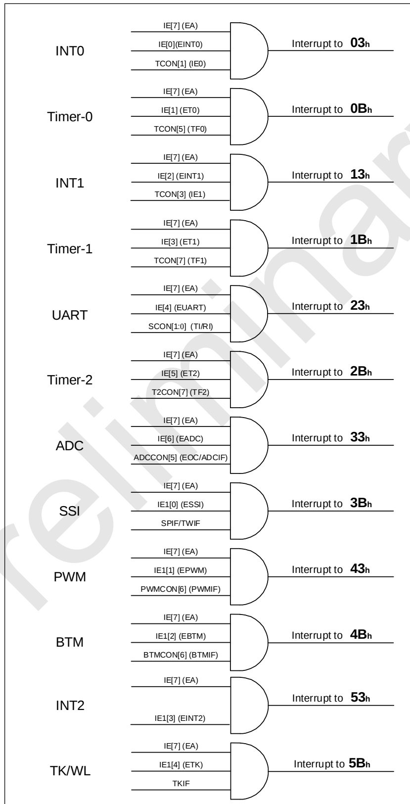
SC92R425 中断结构和向量
