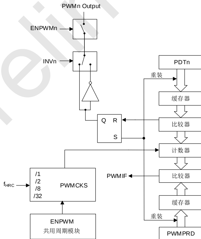
SC92R425 PWM 独立模式框图
