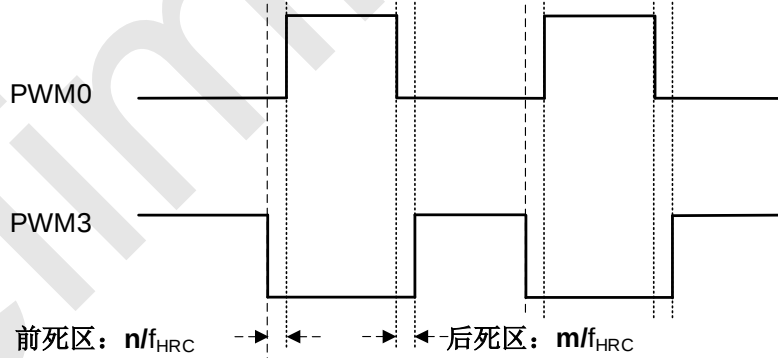
PWM 死区输出波形
