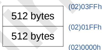
SC92R425 EEPROM Sector 分区示意
