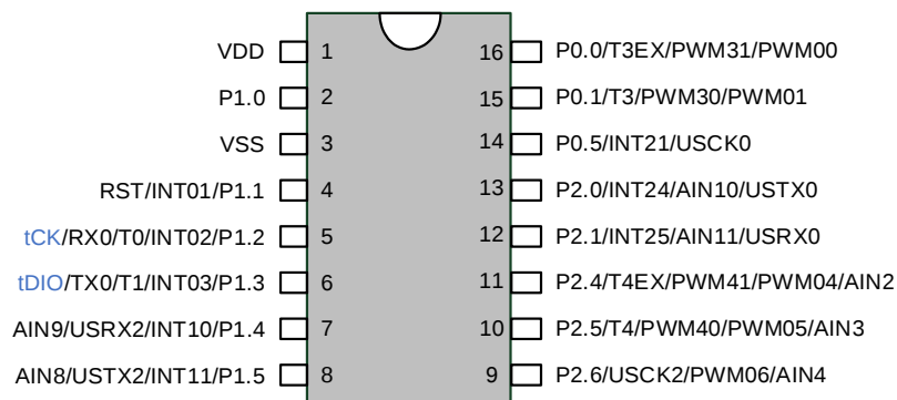
SC95F7571 管脚配置图 适用于 SOP16 封装
