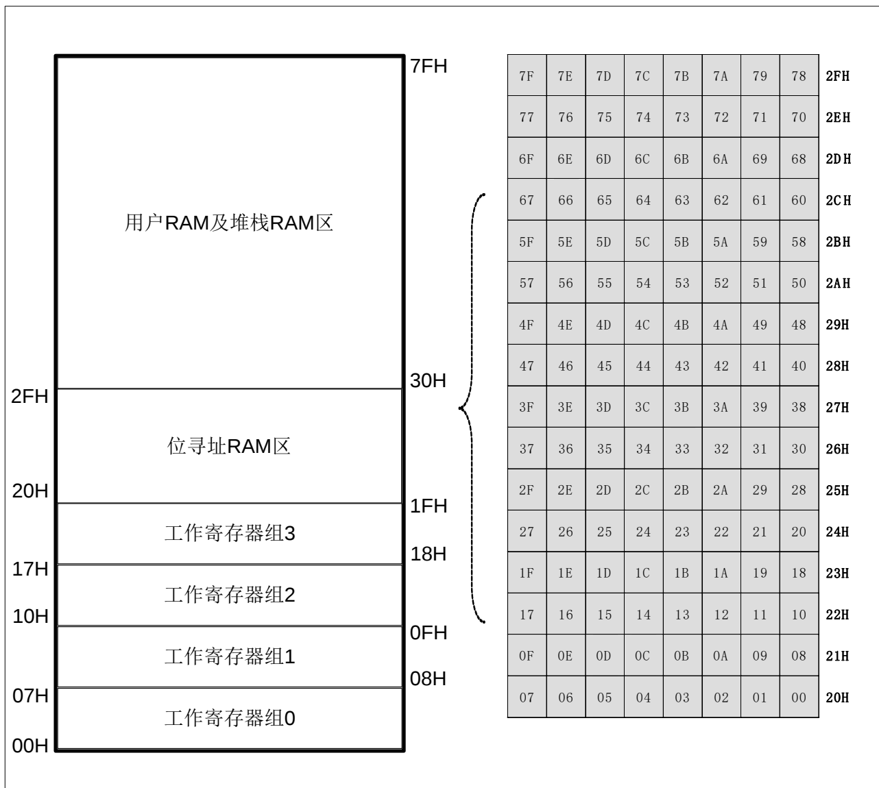
SRAM 结构图
