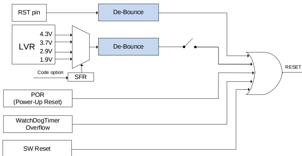
SC95F757X 复位电路图
