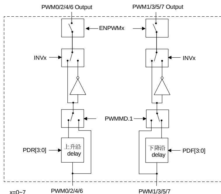
SC95F757X PWM 互补模式框图
