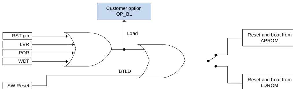
SC95F757X 复位后启动区域切换示意图
