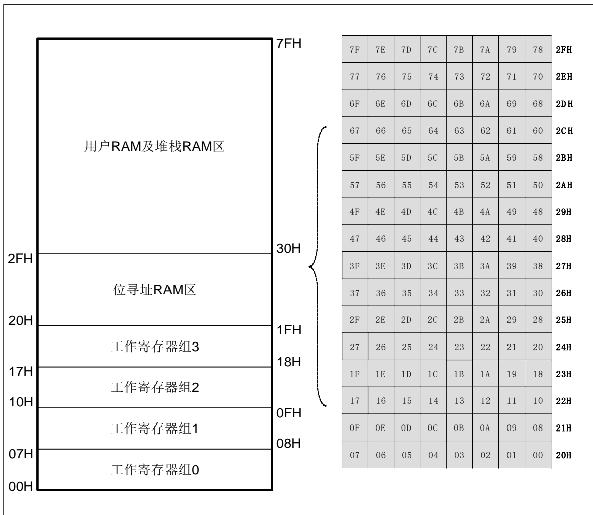
SRAM 结构图
