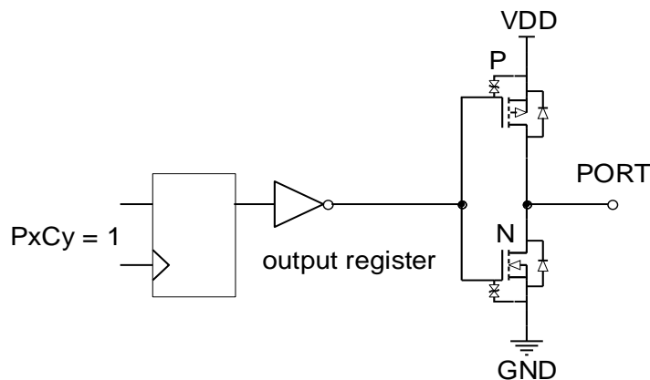
强推挽输出模式
