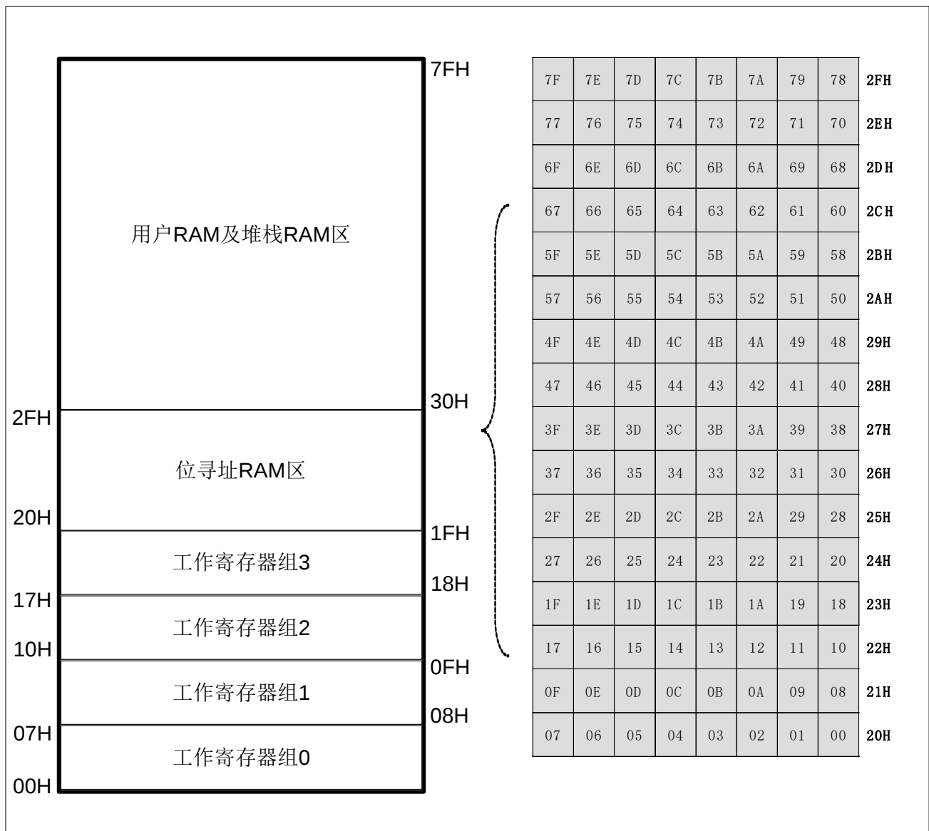
SRAM 结构图
