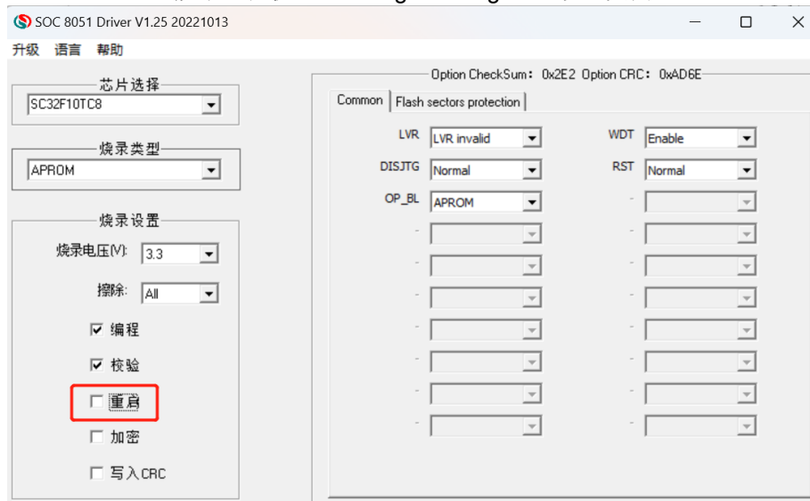
KEIL 插件的设置页面
