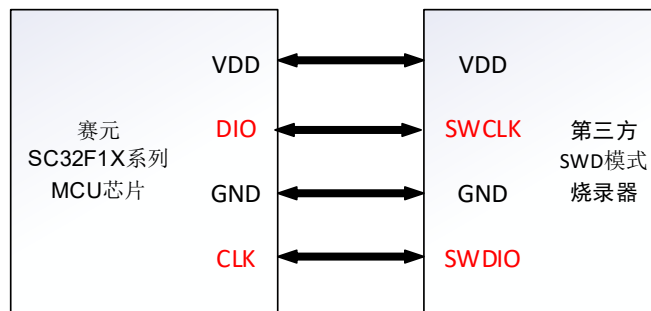
SWD 模式烧录连接图
