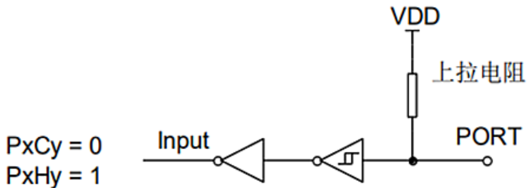
带上拉的输入模式
